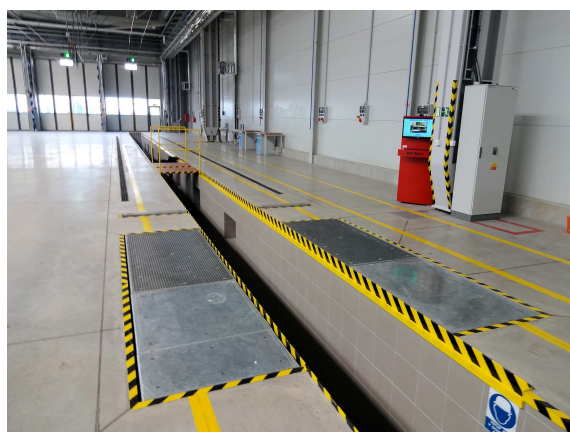
AREX LKW2PSW – zkušebny brzd s testerem sbíhavostí a integrální přejezdovou váhou (nové DEPO Plzeňských městských dopravních podniků ve ŠKODA TRANSPORTATION)
